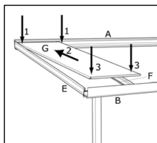
Figur 11 - 12: Tagpladerne "klikkes" på plads.
